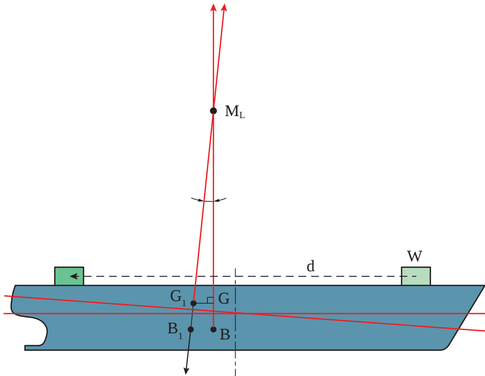
شکل ۱۲- متاسنتر طولی
