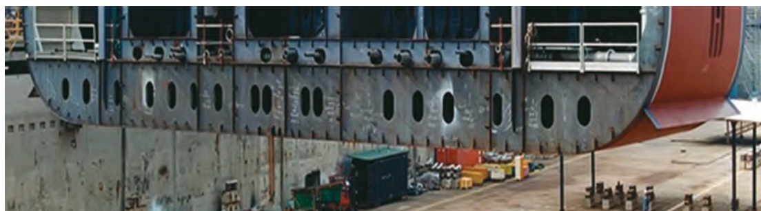
شکل ۱۴- کف دو جداره یک کشتی در حال ساخت
