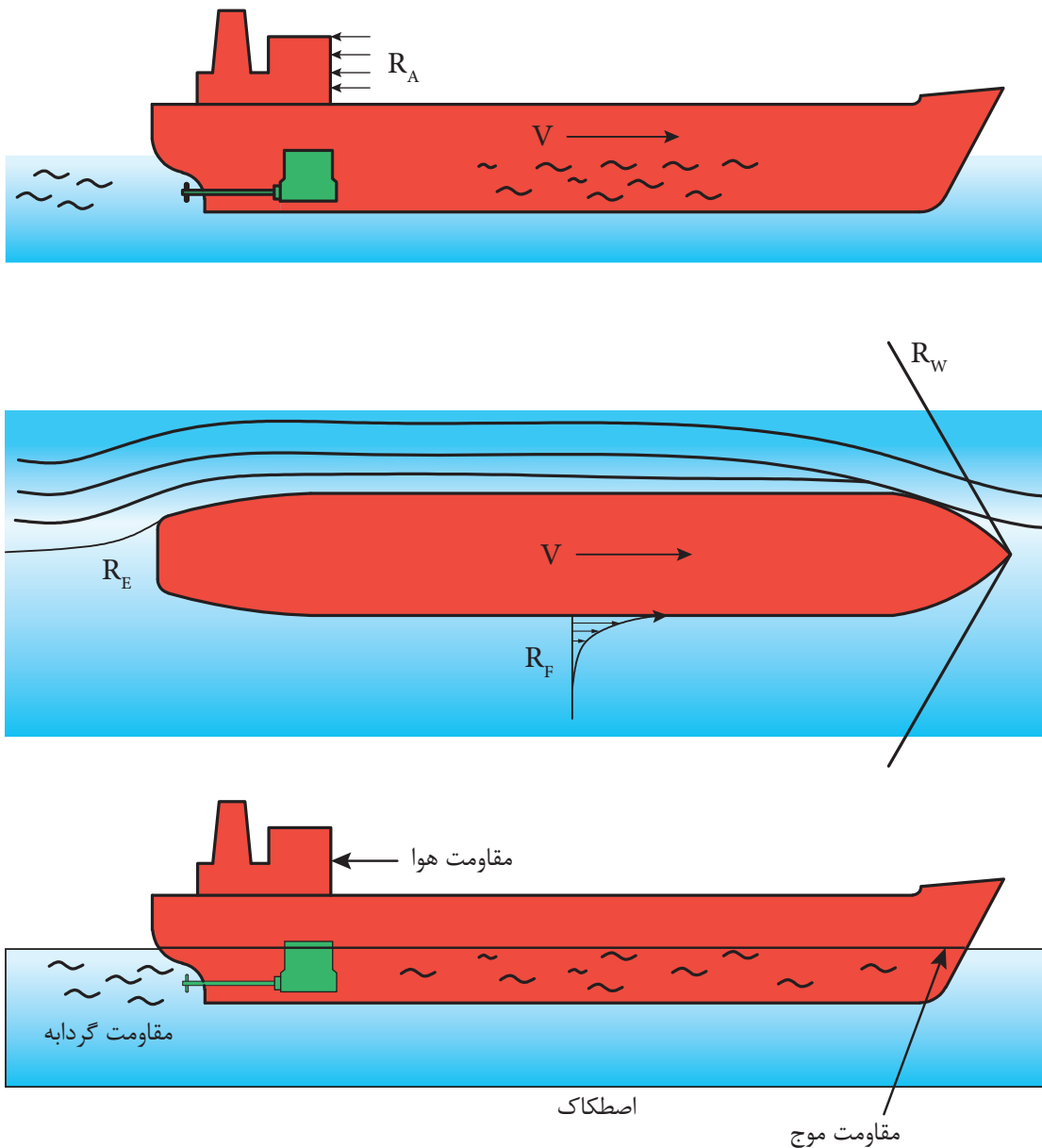
شکل ۷- محل ایجاد نیروهای مقاوم (مقاومت) در برابر حرکت شناور
