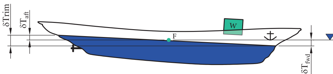
شکل ۱۰- مرکز غوطه‌وری
