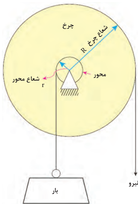
شکل ۲۸- چرخ و محور
