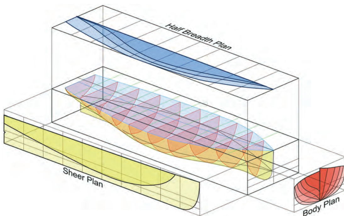
شکل ۲۰ - خطوط بدنه در مقاطع مختلف
