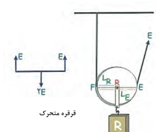
شکل ۲۵- قرقره متحرک
