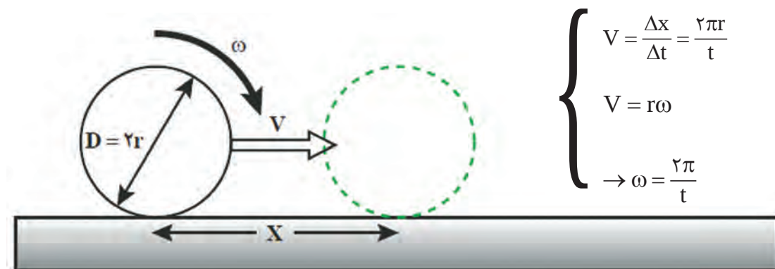
شکل ۱۴- جابه جایی مرکز جرم در اثر دوران
